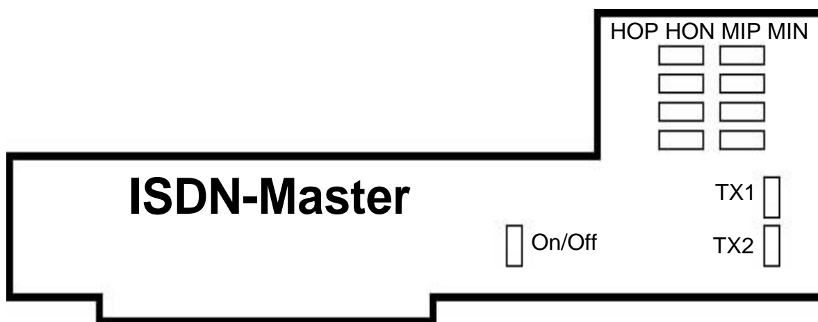
Anordnung der Steckbrücken
