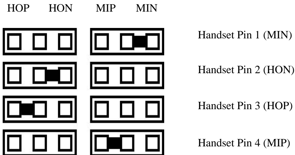
Die Steckbrückenmatrix des Telefonhöreranschlusses
